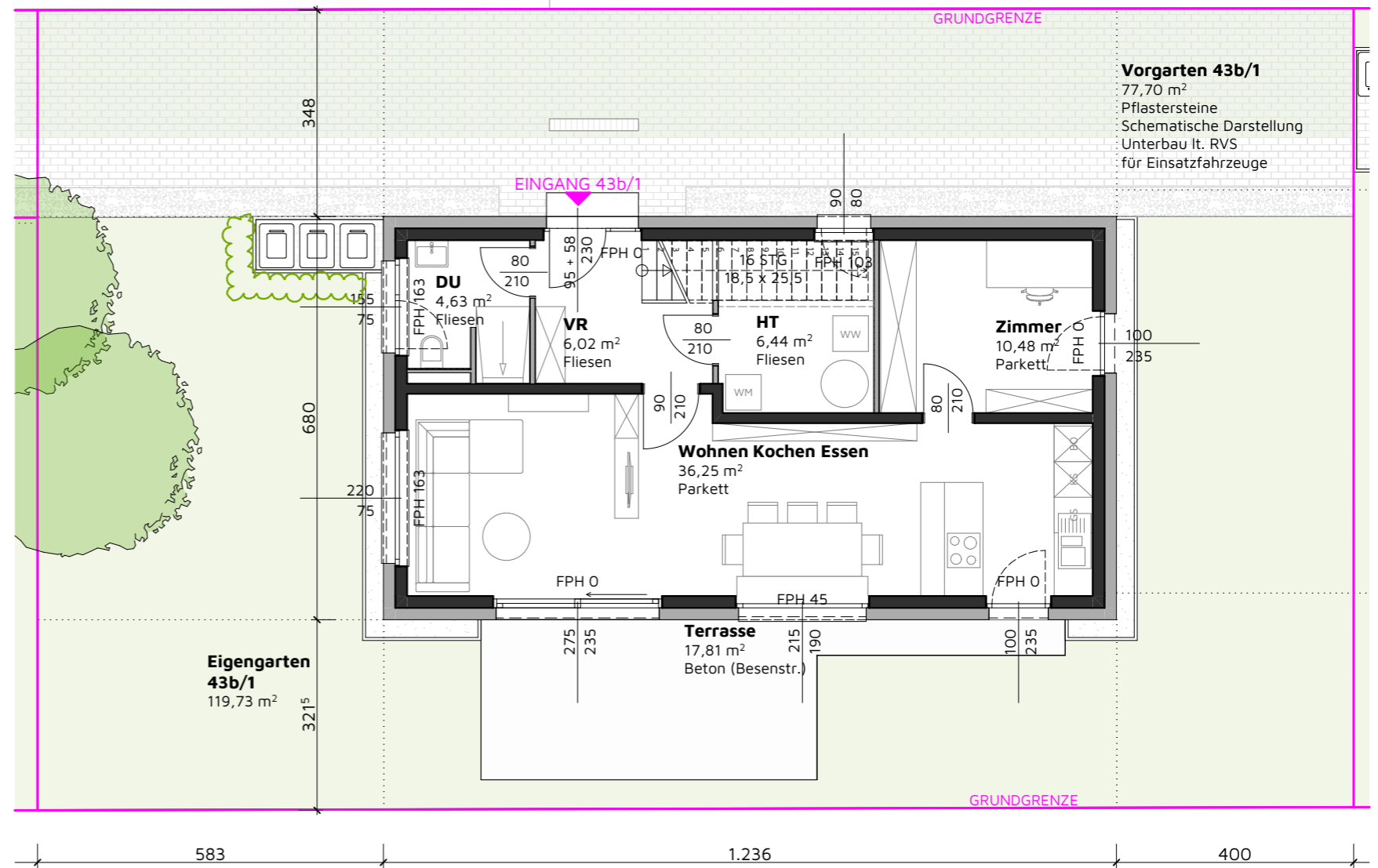
0. Erdgeschoss 1:100
