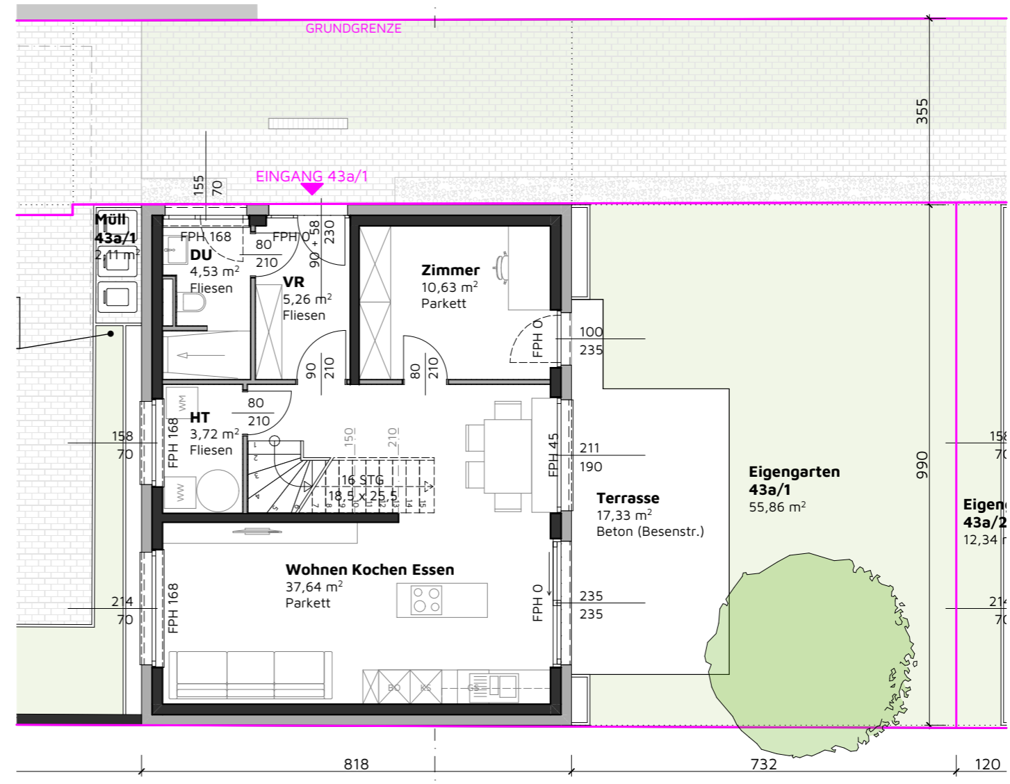
0. Erdgeschoss 1:100
