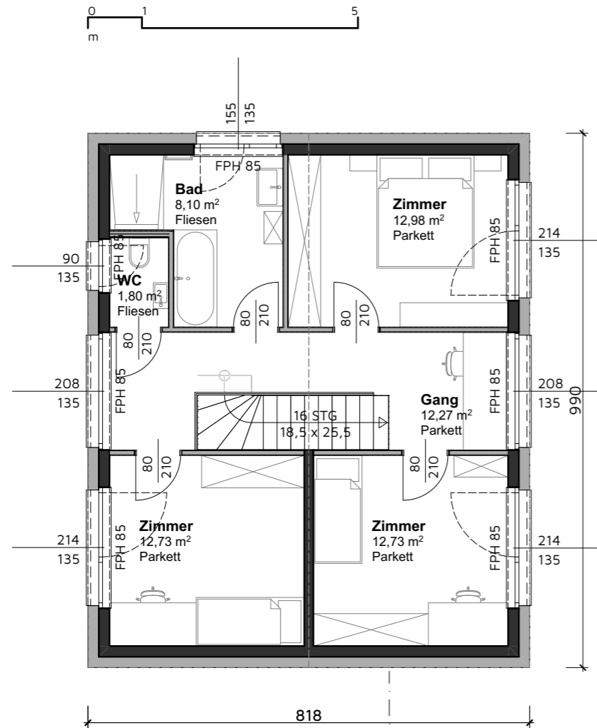
1. Obergeschoss 1:100
