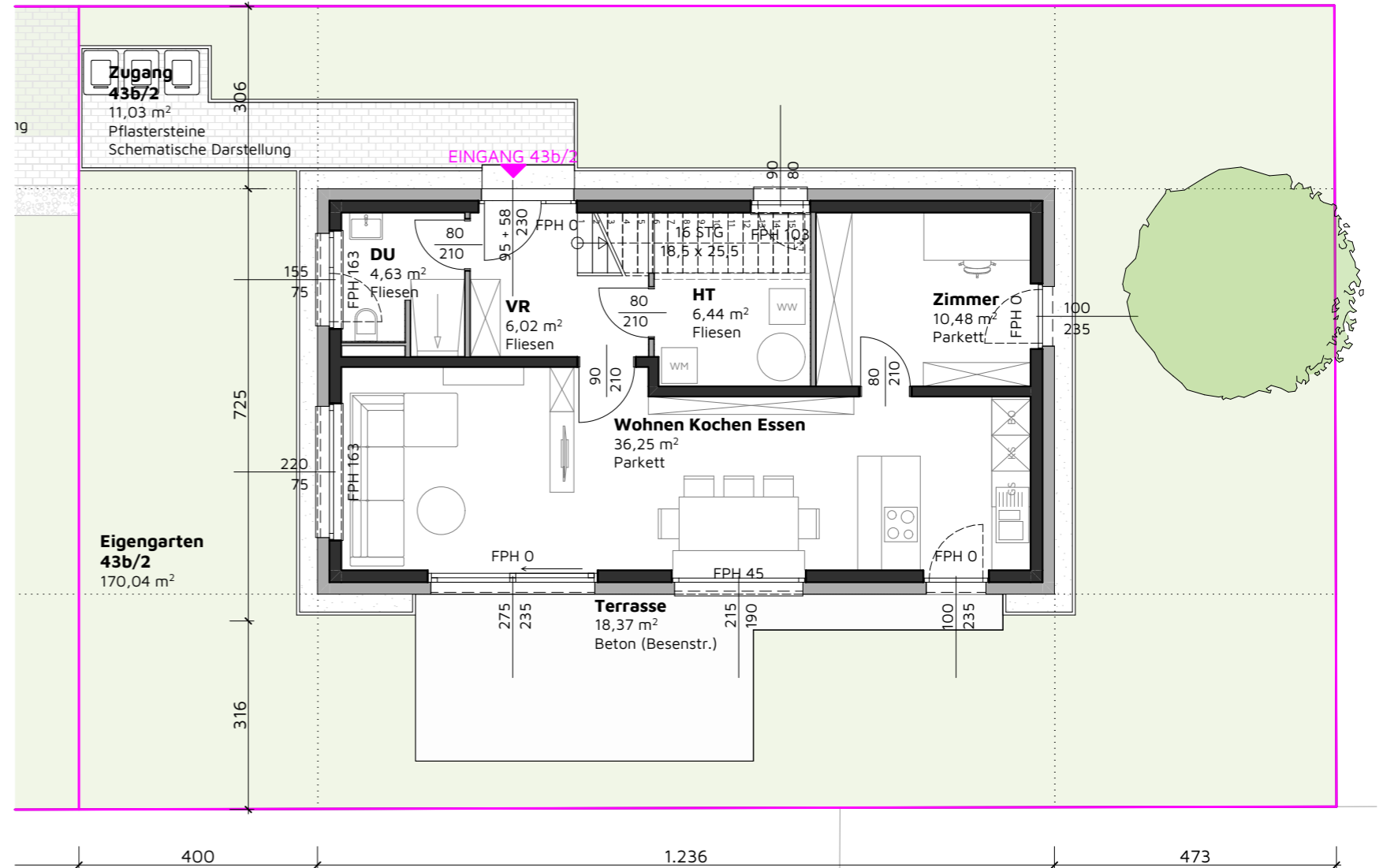
0. Erdgeschoss 1:100
